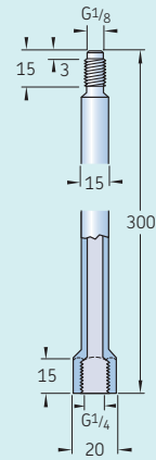
Tubo de extensão G 1/8
