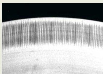
Marcas de estrias características da erosão elétrica em rolamentos
