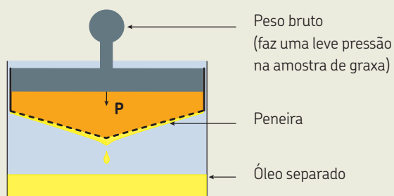
Teste de separação de óleo
