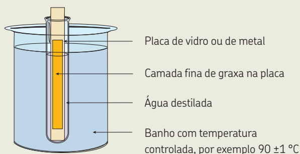
Teste de resistência à água
