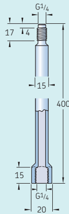
Tubo de extensão G 1/4
