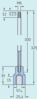
Tubo de extensão M6 com niple de conexão
