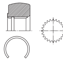
Trava intermediária
